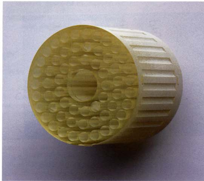
Das nach dem stereolithografischen Modell hergestellte Bauteil aus ABS (oben) war zu ungenau und zu schwer. Das fertigungsgerechte Konstruieren einer Baugruppe war zwar eine technische Herausforderung, verhalf aber der Erfindung zum Durchbruch.
